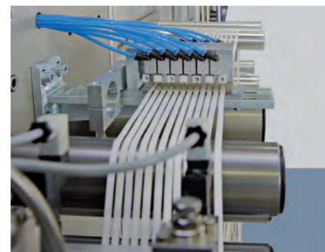
Pneumatische Streifenbremse
