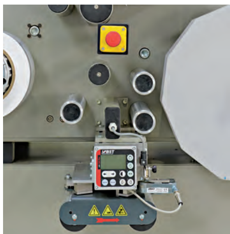
Bahnlaufregelung
